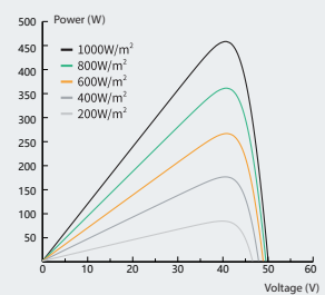
Power-Voltage Curve(455W)
